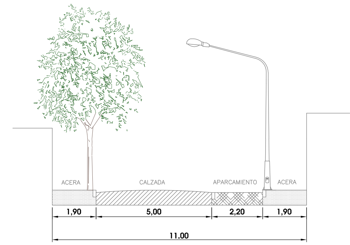
SECCIÓN TIPO B-B' COTAS en Metros ESCALA: 1/100
